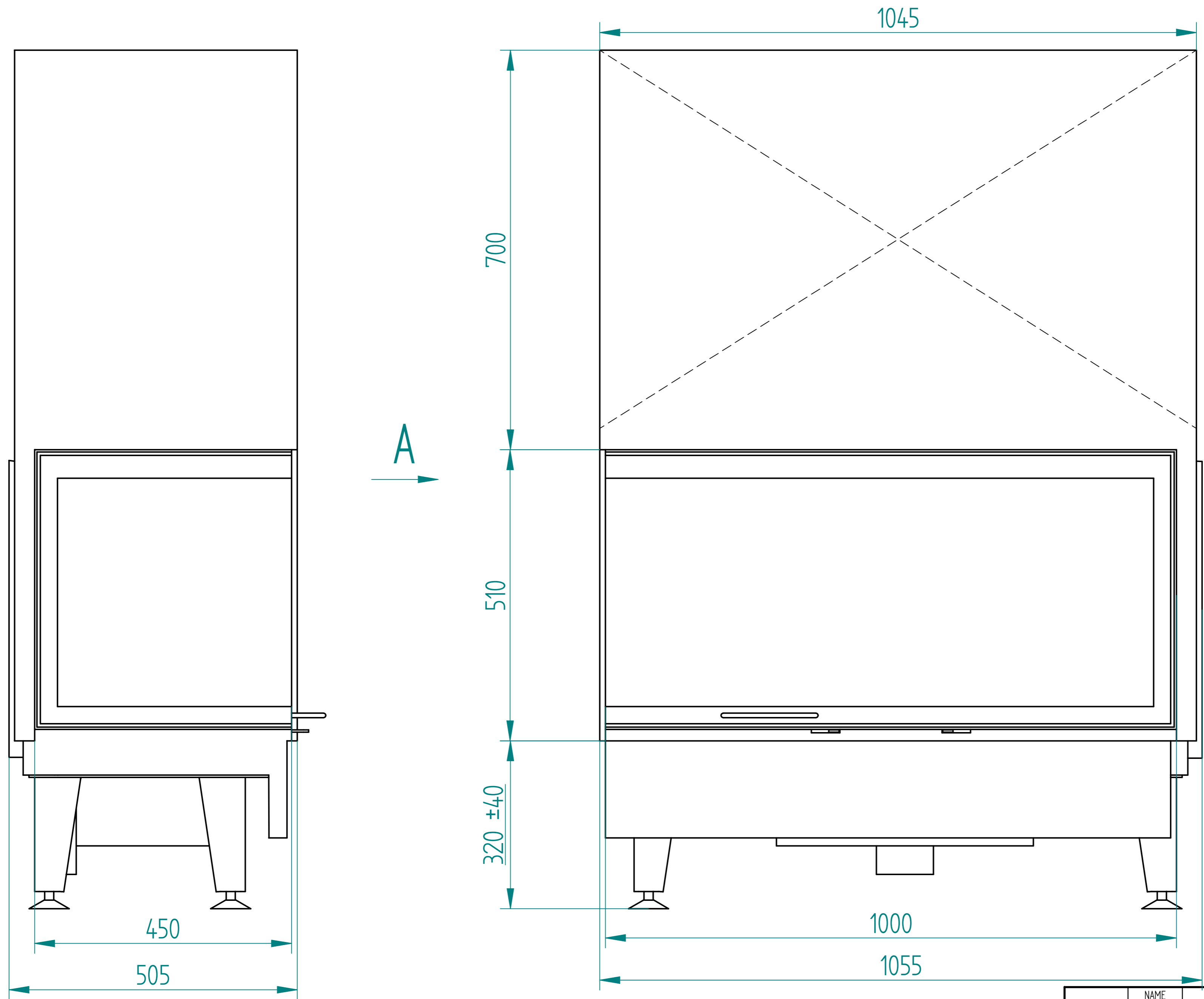
Widok A
