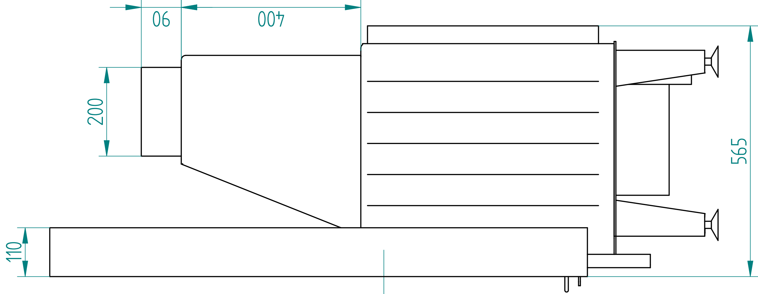
Widok A
