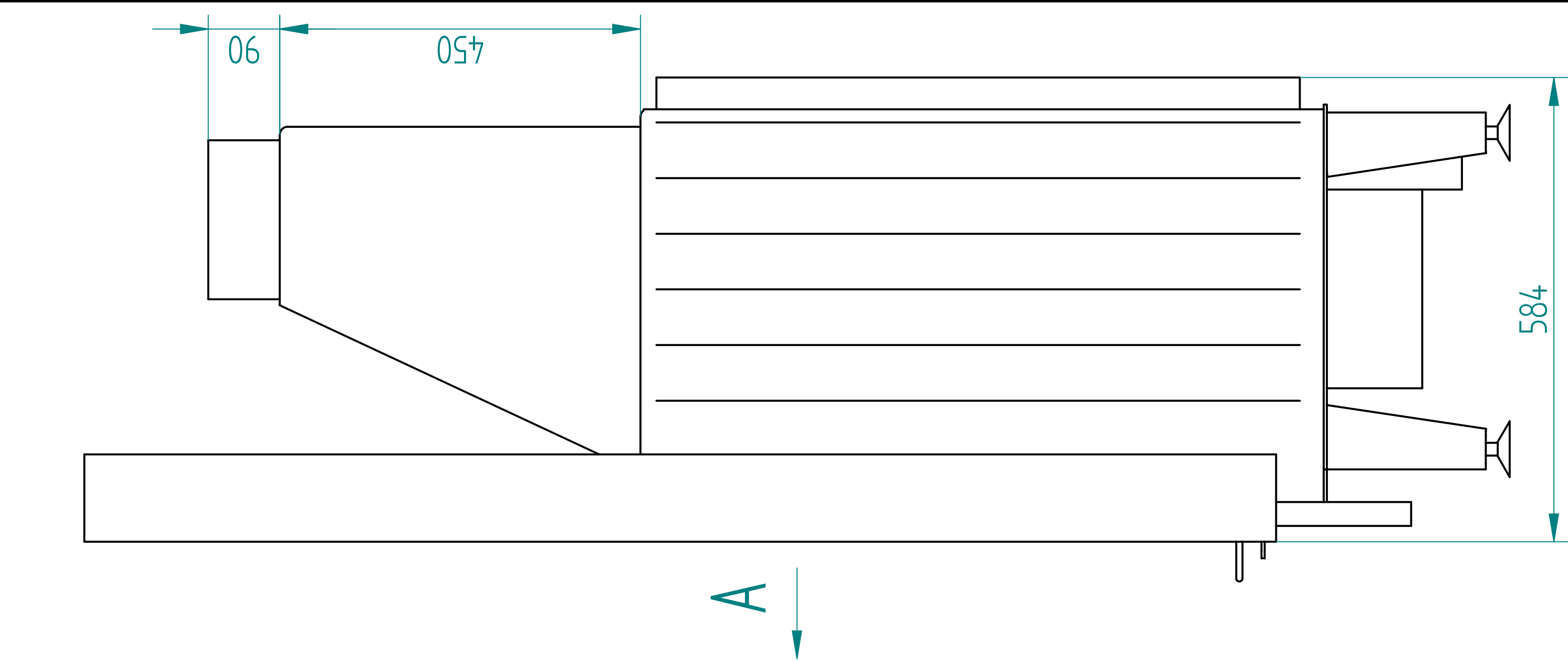
Widok A
